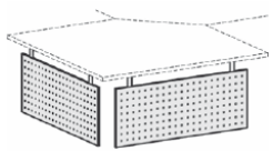
Knieraumblende gelocht für Fünfeck-Platte Höhe 400 mm
