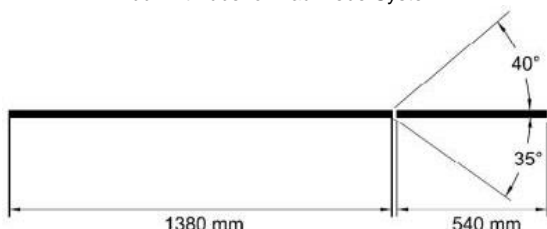
Abb. mit Zubehör Rad-Hebe-System
