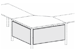
Knieraumblende für Fünfeck-Platte, mit Montage-Set Höhe 475 mm
