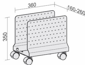
Mobiler CPU-Halter mit Lochblech- Seitenteilen, inkl. 4 Rollen
