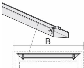
Kabelkanal abklappbare Kabelhalbschale
