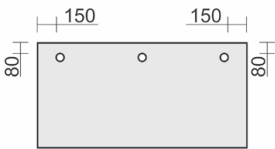
Kableinlassbuchse D: 60 mm wählbare Dekore: L - Lichtgrau Z - Schwarz S - Silber
