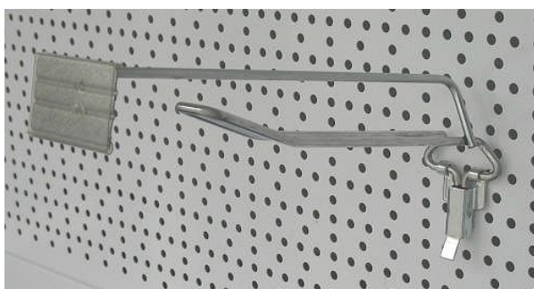
Doppelhaken mit Schild 60 x 44 mm und Scanning Clip Profil verzinkt, für Lochabstand 15 mm.
