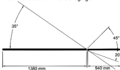
Abb. mit Zubehör: Extensionsgalgen
