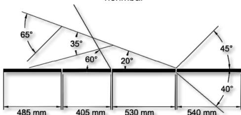
Negativlage bei Option 3-teiliges Kopfteil max. -30°
