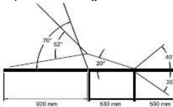
Negativlage bei Option 3-teiliges Kopfteil max. -30°
