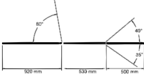
Negativlage bei Option 3-teiliges Kopfteil max. -30°
